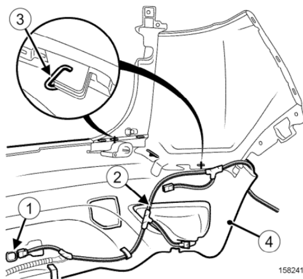
جزئیات مکانیزم درب جانبی
