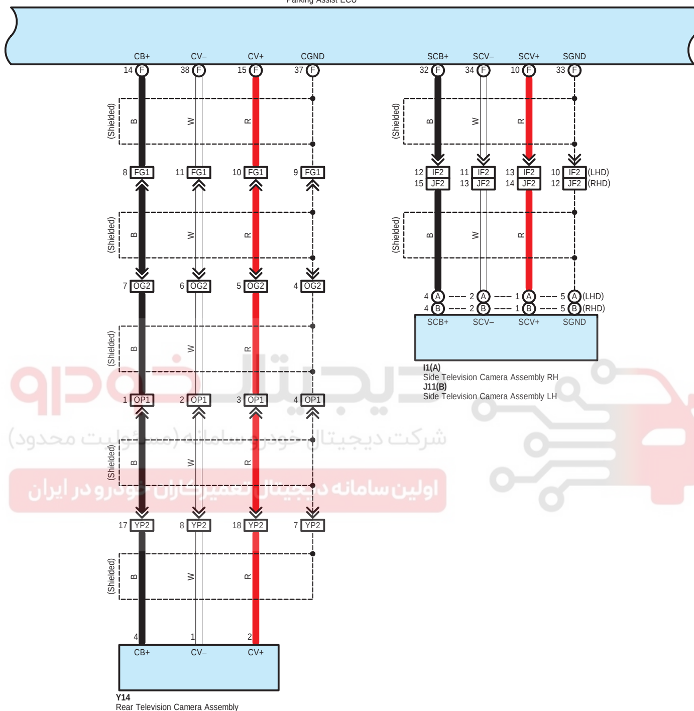
F103(E), F104(F), F106(G) Parking Assist ECU
