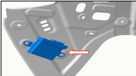
طرح کلی ماژول کنترل رادار دنده عقب (بر روی صفحه پشت سینی عقب چپ)
