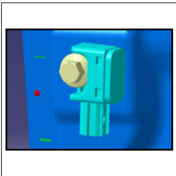
حسگر برخورد جانبی (روء صفحه فلزء ستون وسط (B) در دو طرف)
