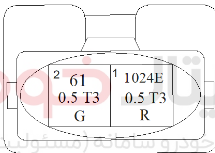
کانکتور توربو
