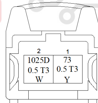
کانکتور انترکتور
