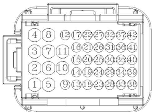
کانکتور دسته سیم داشبورد به دسته سیم موتور
