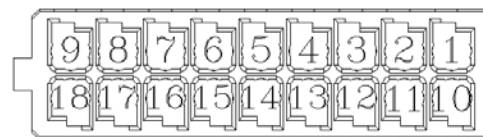
کانتور صفحه کیلومتر پشت آمپر
