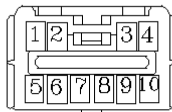
کانکتور دسته سیم عقب راست به دسته سیم درب عقب
