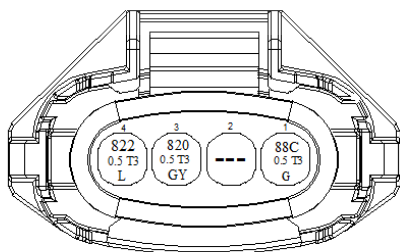
کانکتور سنسور بوست
