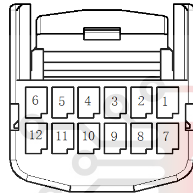
کنکتور کلید استارت استپ
