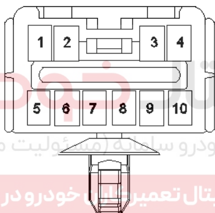
کانکتور دسته سیم داشبورد به دسته سیم اصلی
