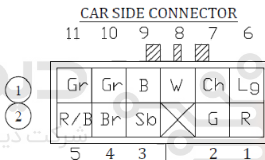
کانکتور ارتباطی بین دسته سیم داشبورد و دسته سیم HVAC CON (AC)
