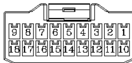
کانکتور دسته سیم عقب چپ به دسته سیم داشبورد 1
