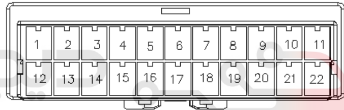
کانکتور دسته سیم اصلی به دسته سیم داشبورد 2
