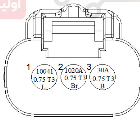
کانکتور برق کوئل
