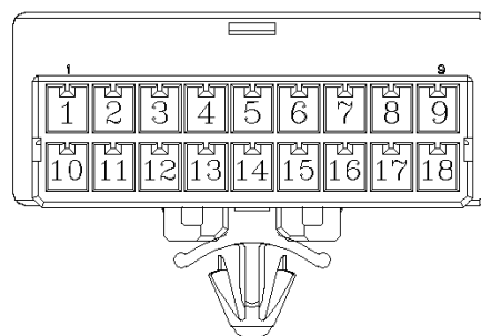
کانکتور دسته سیم داشبورد به دسته سیم چپ عقب 1
