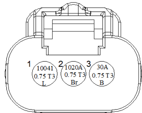
کانکتور برق کوئل
