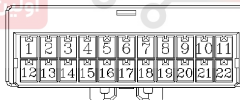
کانکتور دسته سیم داشبورد به دسته سیم عقب راست
