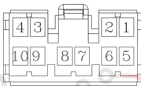
کانکتور دسته سیم عقب چپ به دسته سیم سپر
