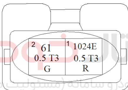
کانکتور توربو
