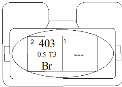
کانکتور سنسور فشار روغن
