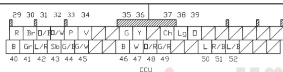
کانکتور کنترل دیجیتال تهویه مطبوع CCU
