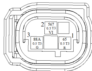
کنکتور سنسور دما
