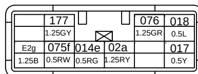
Left front door (30-I)
