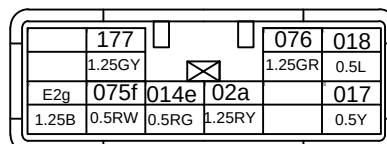
Left front door (30-I)
